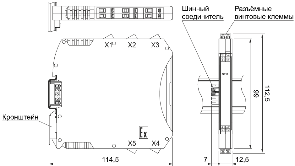
Рисунок 6.1 – Габаритные размеры барьера KA5013Ex-NN
