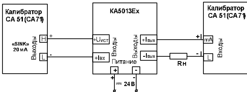
Рисунок 6.4.1А – Подключение барьеров мод. КА5013Ех для поверки преобразования входных унифицированных сигналов постоянного тока (входной пассивный сигнал) в диапазоне от 4 до 20 мА в выходной унифицированный сигнал постоянного тока от 4 до 20 мА
