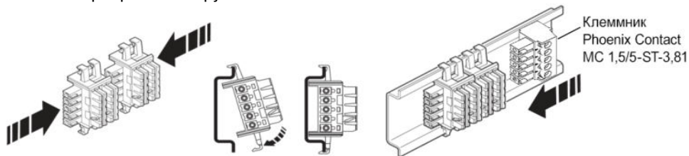
Рисунок 6.3 – Установка шинных соединителей на DIN- рейку
